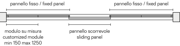
Composizione lineare Linear composition
