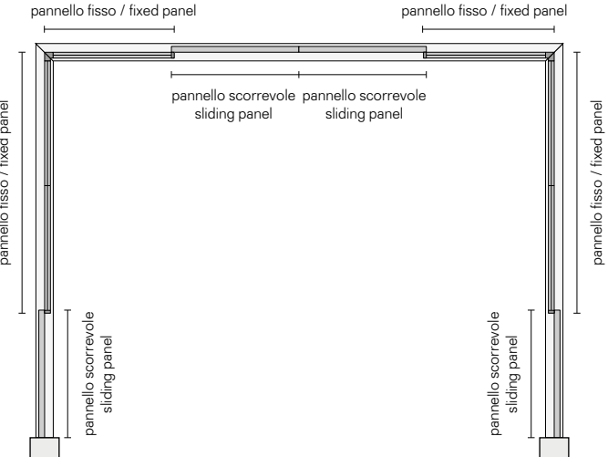
Composizione articolata Modular composition
