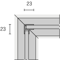
Montante angolare Corner joint
