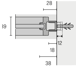
Telaio a pavimento con regolazione telescopica Floor frame with telescopic adjustment
