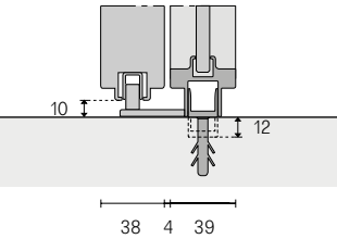
Sistema di fissaggio a terra con regolazione di 12 mm Floor fixing system with 12 mm adjustment
