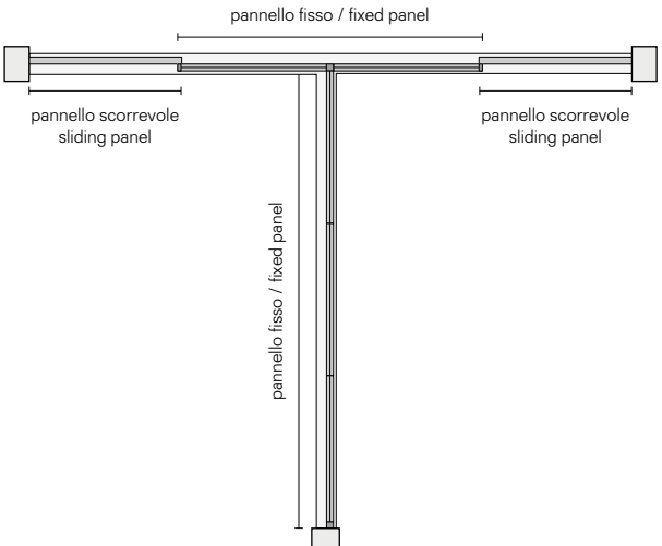
Composizione a T T-shaped composition
